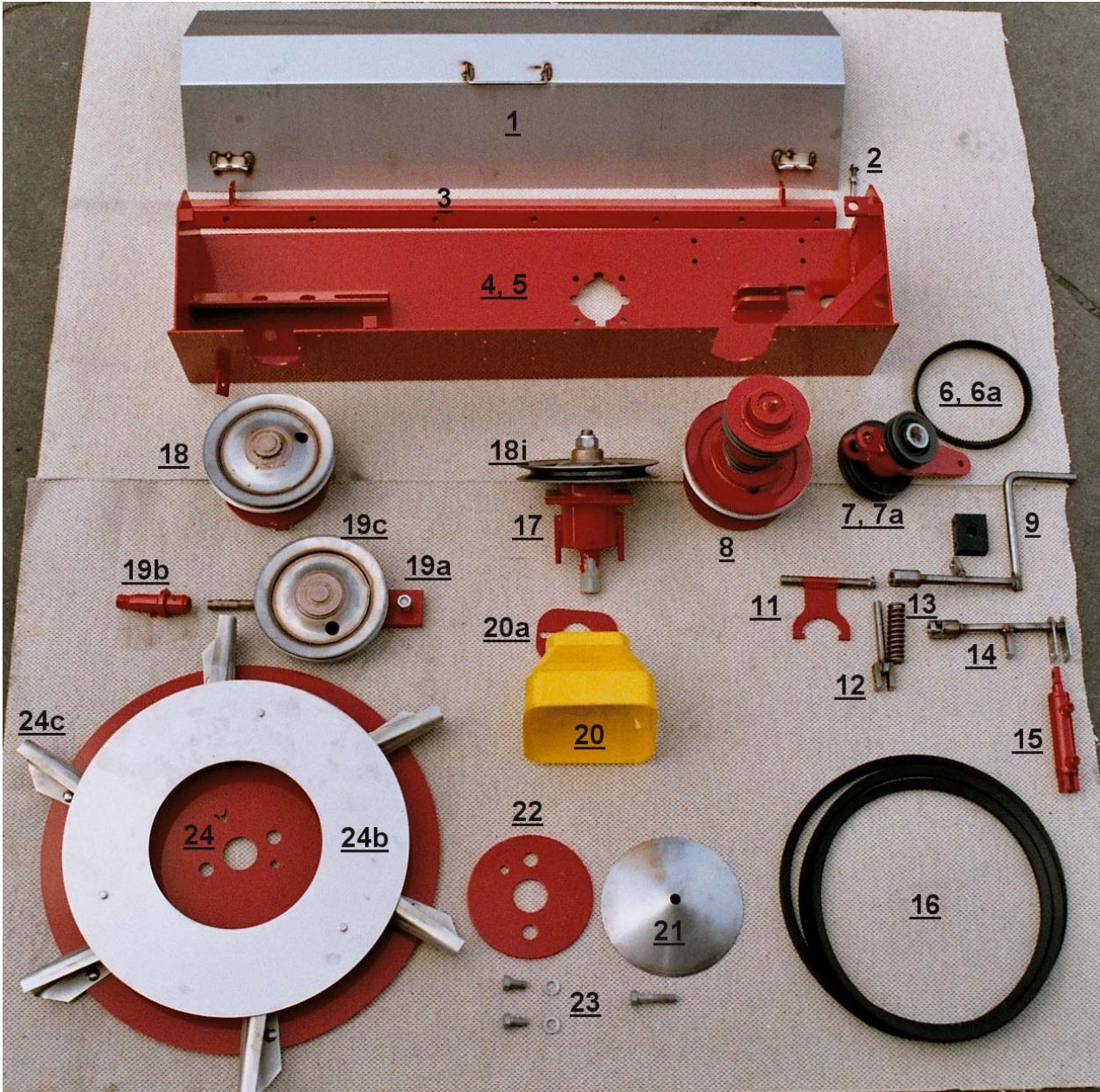
Spredkasse SPC4500-1 med kantgear / spread box SPC4500-1 with headland gear / Streuwerk SPC4500-1 mit Grenzstreugetriebe
